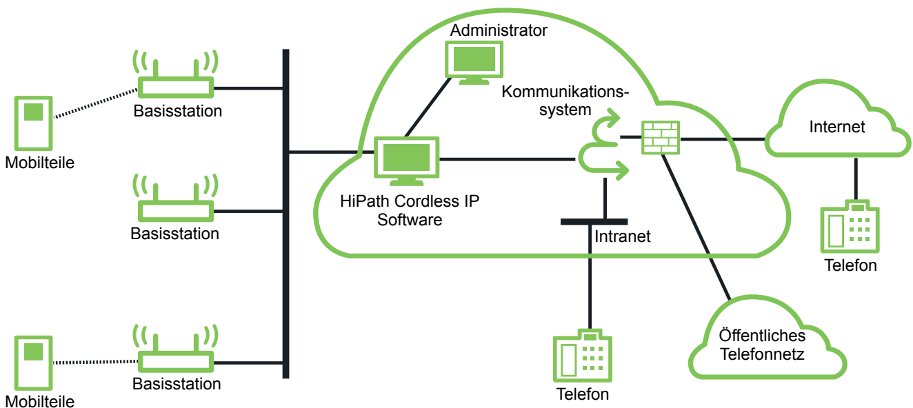
Konfiguration/Systemkonzept
