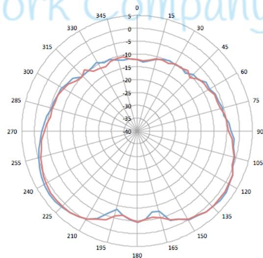
5.5GHz Wi-Fi (antennas A,B,C,D)
