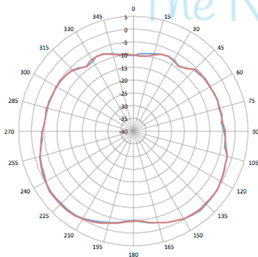
2.45GHz Wi-Fi (antennas 1,2,3,4)
