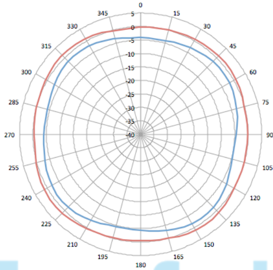
2.45GHz Wi-Fi (antennas 1,2,3,4)
